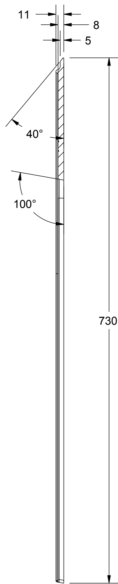
SECTION A-A
